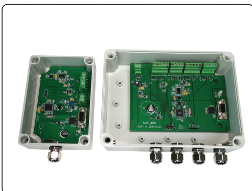
[Board 조립사진]
