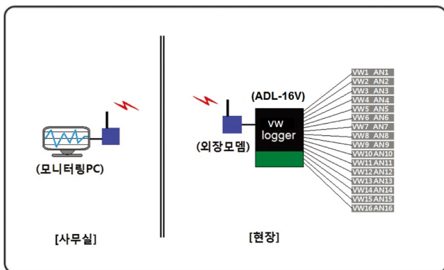
[ADL-16V 시스템 구성도]
