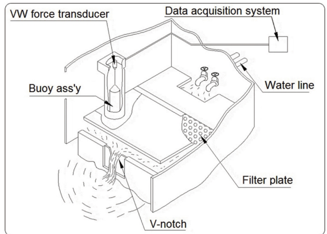
[진동현식 수위 측정 시스템 설치도]
