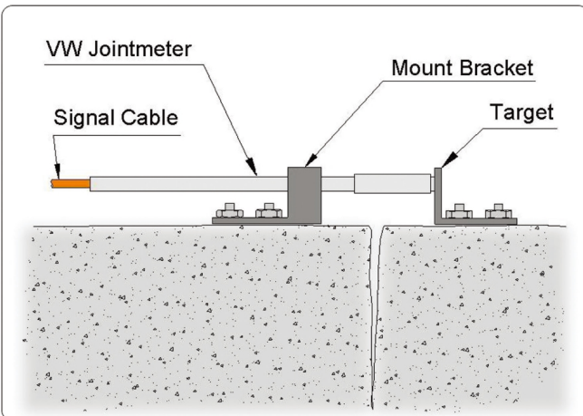
[진동현식 압축형 변위계 설치도]
