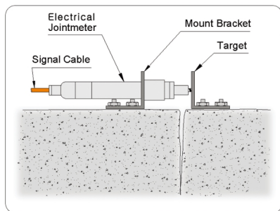
[단축 설치도]
