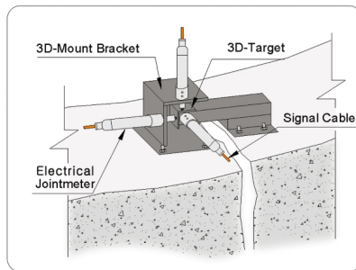
[3축 설치도]
