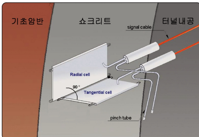
[진동현식 쇼크리트 응력계 설치그림]
