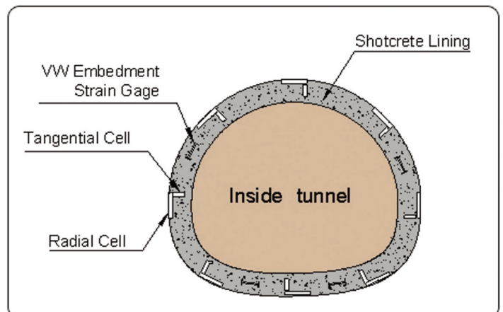
[진동현식 쇼크리트 응력계 설치 단면도]
