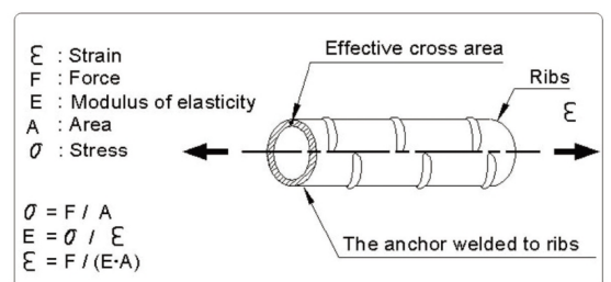
[계산 이론]
